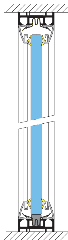
Coupe verticale
