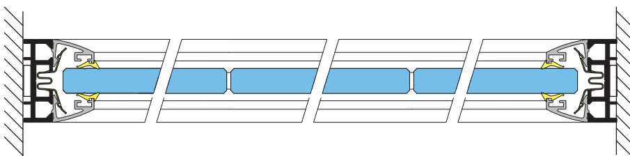
Coupe horizontale
